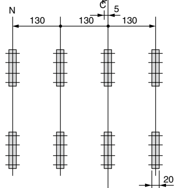
Вертикальное подсоединение
