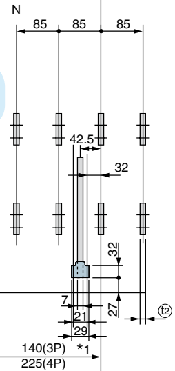
Вертикальное подключение
