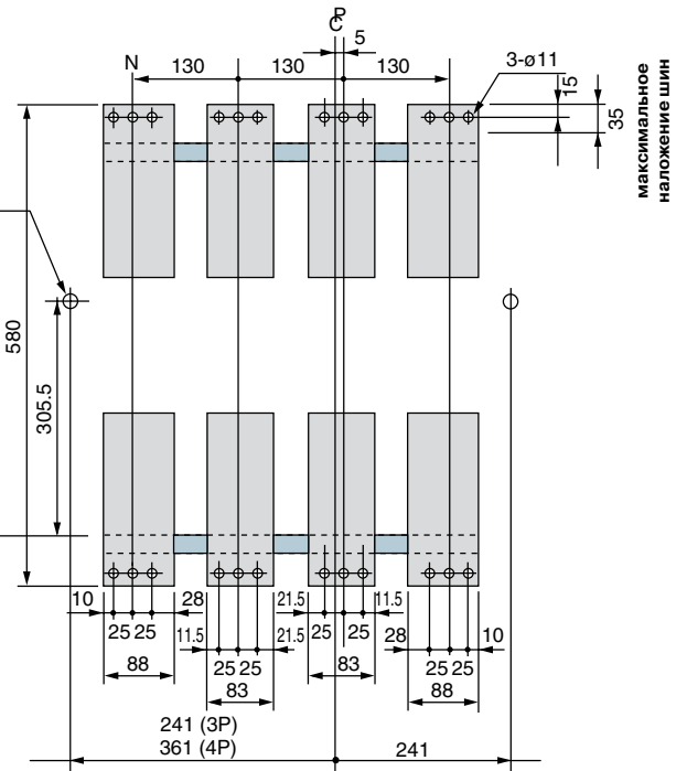
Вертикальное подсоединение
