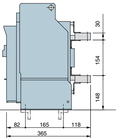
Горизонтальное подсоединение
