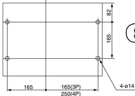
Монтажные отверстия
