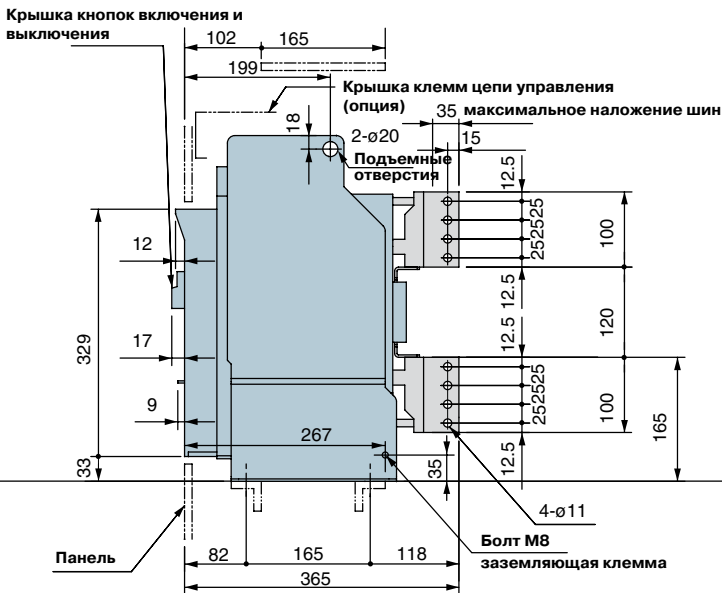
Вертикальное подсоединение
