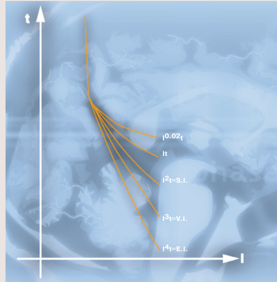
Время-токовые характеристики: зависимость времени срабатывания расцепителя от значения сверхтока
